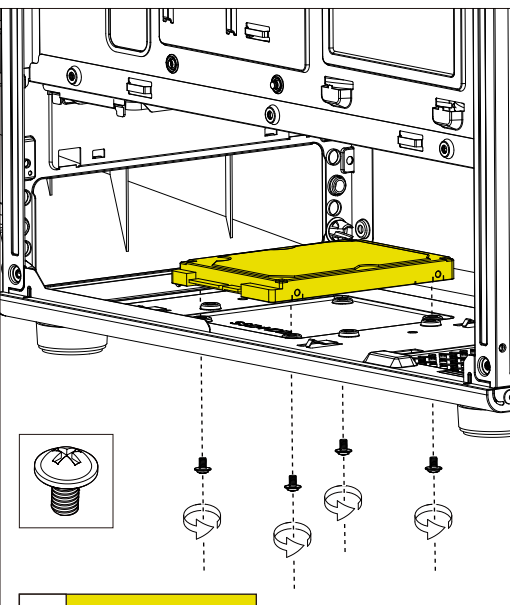
C2 Bottom 2.5" SSD
