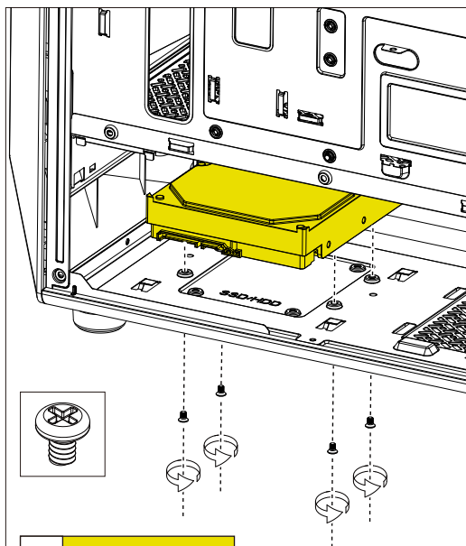
C1 Bottom 3.5" HDD
