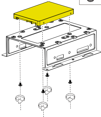
A3 Top Single 2.5" SSD
